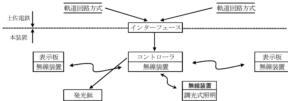
図3 ノーガード電停安全対策システム構成
