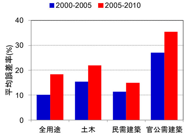
図-13 最近10年間の生産年齢1人当りのコンクリート増加率の平均誤差率の各用途間の比較（含沖縄県）
