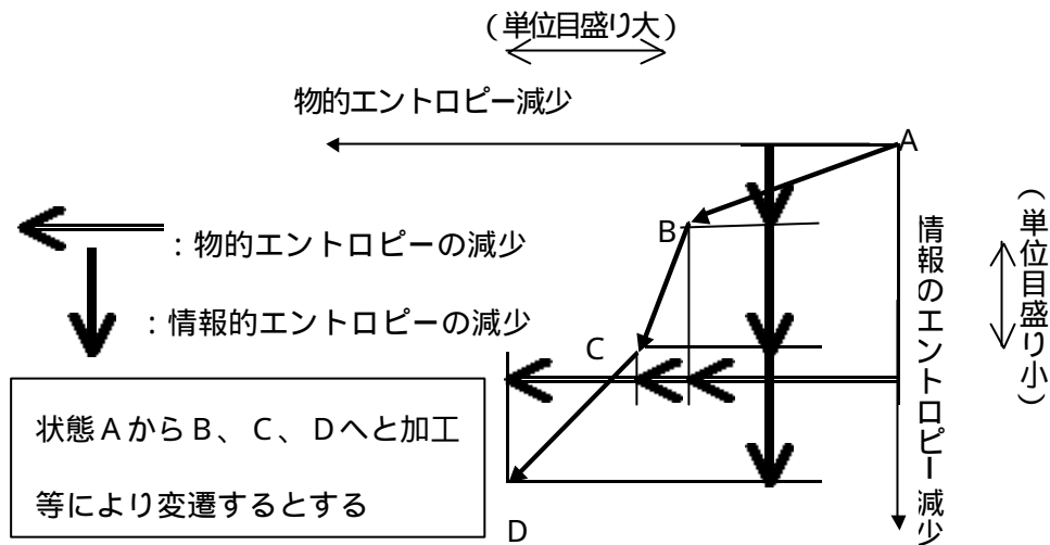
図2 - 3 状態間のエントロピーの減少
