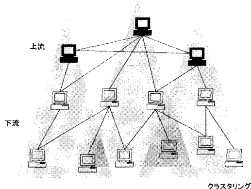
図 1 Winny における階層構造とクラスタリング
